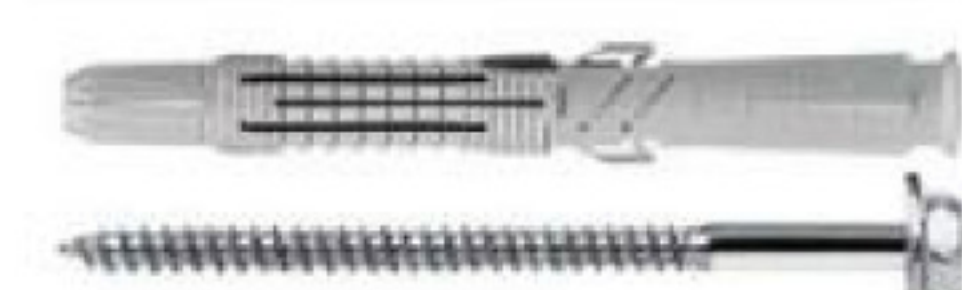
Анкер PROLONGI-H / T88-H + винт с шестигранной головкой
